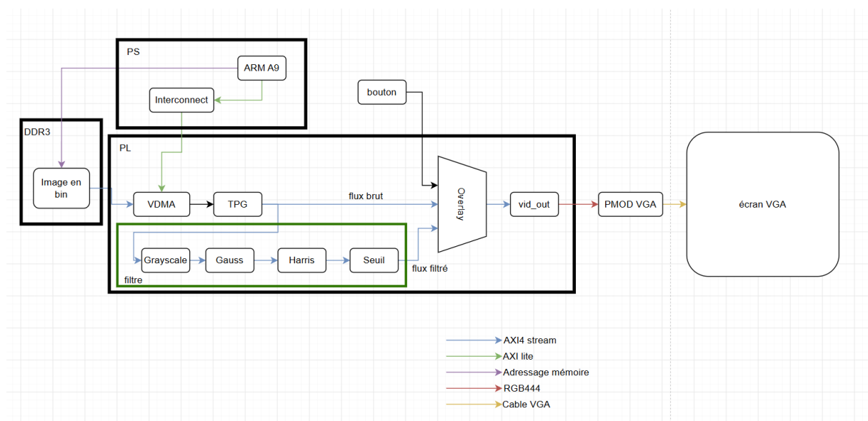
FIGURE 1 : SCHEMA SYNOPTIQUE
