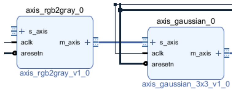
FIGURE 5 : BLOC IP GRAYSCALE ET FILTRE DE GAUSS
